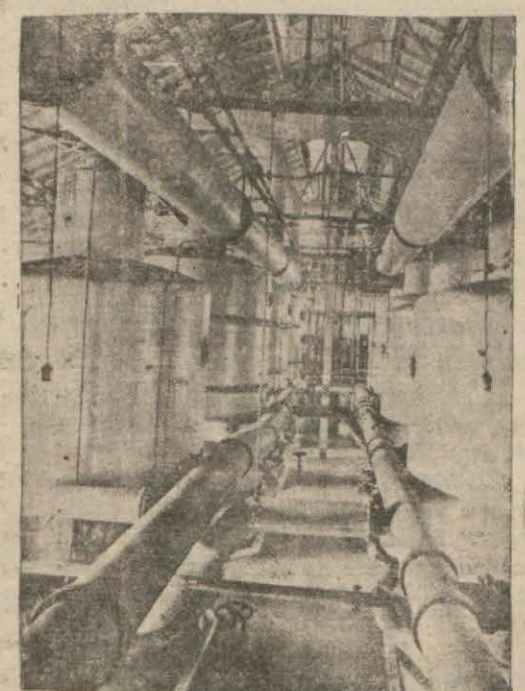
Şeker fabrikalarından birisinin muazzam istihsal cihazları
