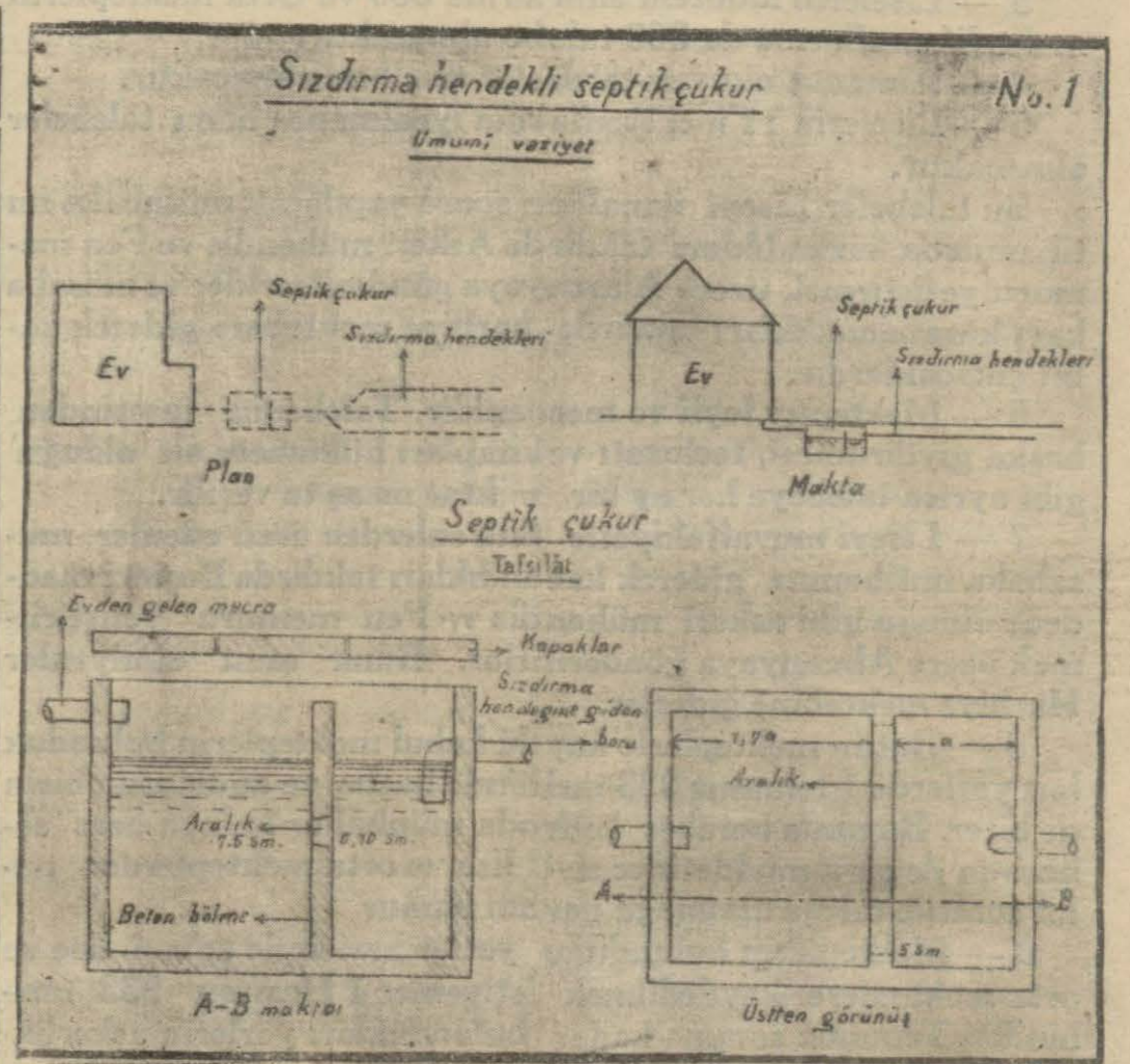
Sızdırma hendekli septik çukur
