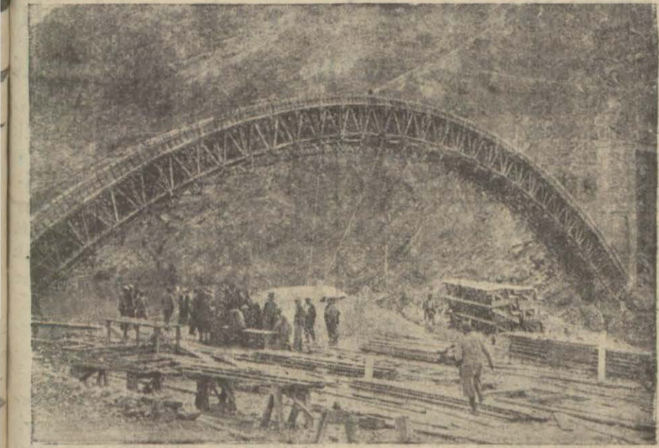
Fıratta Komürhanda 160 metrelik Şose köprüsü
