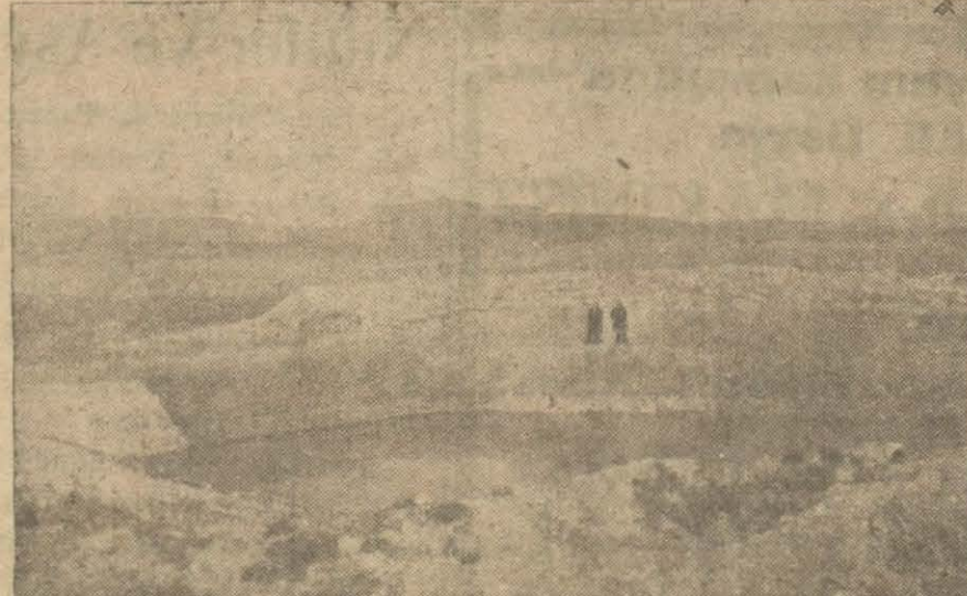
Ahmesutla Ankara arasında Tahar denilen köy civarında yer altı sularının toplanmasına mahsus bunnık bir bent yapılmıştır. Bendin hacmi 4500 metre mikabidir. Bent bir kapakla boşaltılabilmektedir.
